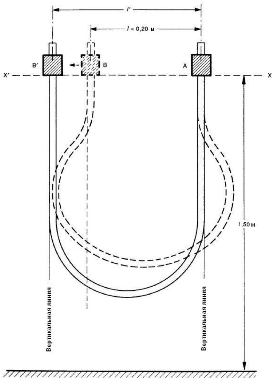
Рисунок 3 – Испытание на статическую гибкость
