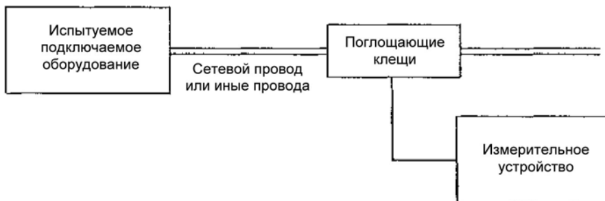
Рисунок 10 – Схема для измерения мощности помех от подключаемого оборудования (за исключением видеомагнитофонов) (см. 5.6.3)
