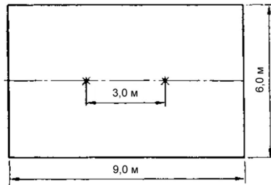
Рисунок 11 – Измерительная площадка (см. 5.7.2)
