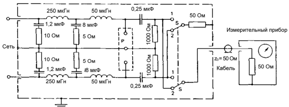
Рисунок 4 – Пример эквивалента сети 50 Ом – 50 мкГн – 5 Ом (см. 5.3.1)
