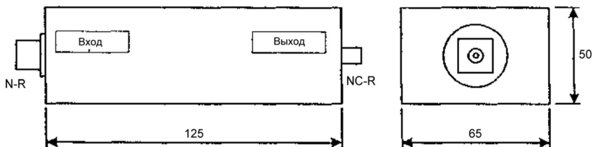
Рисунок А.3 – Типовые размеры изолирующего трансформатора для диапазона частот от 46 МГц до 1,5 ГГц
