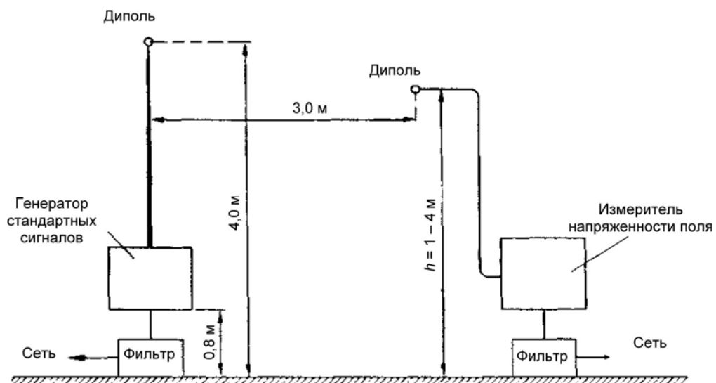
Рисунок 12 – Проверка соответствия измерительной площадки (см. 5.7.2)
