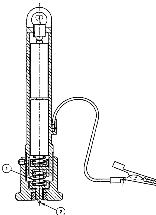
1 – пружина с усилием нажатия 10 Н; 2 – наконечник, которым производится царапание (стальной шарик диаметром 1 мм)
