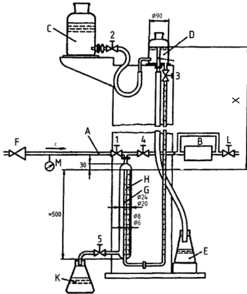
А – вход; В – испытуемый образец; С – емкость для воды; D – сосуд с постоянным уровнем воды; E – переливной сосуд; F – регулятор давления; G – трубка; H – измерительная бюретка; K – сливной сосуд; L – кран на выходе; 1-5 – ручные краны
