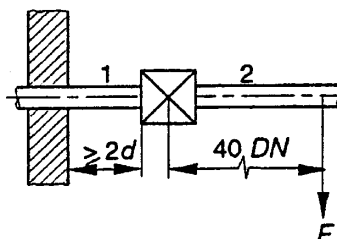
Рисунок 2 — Схема сборки для испытания изгибающим моментом
